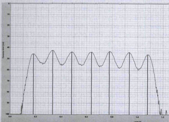
Rys. 5. Obraz raportu skanu urządzeniem Lithoscope ze zbrojeniem o średnicy 12 mm
